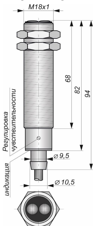
Габаритный чертеж
