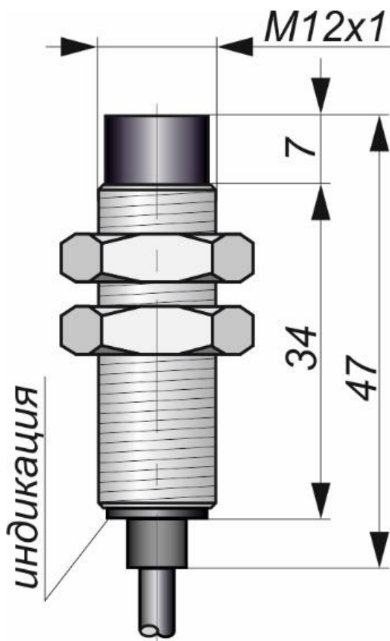
Габаритный чертеж
