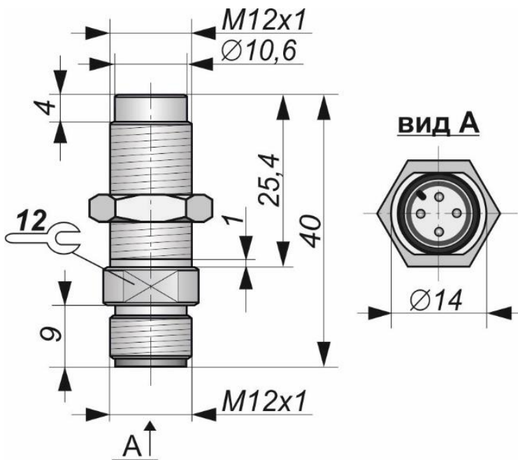
Габаритный чертеж
